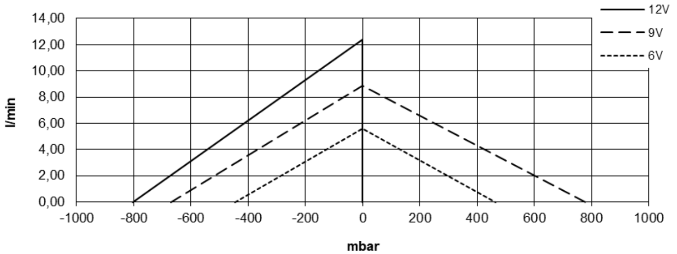
Type/Model: DC12/90KL
