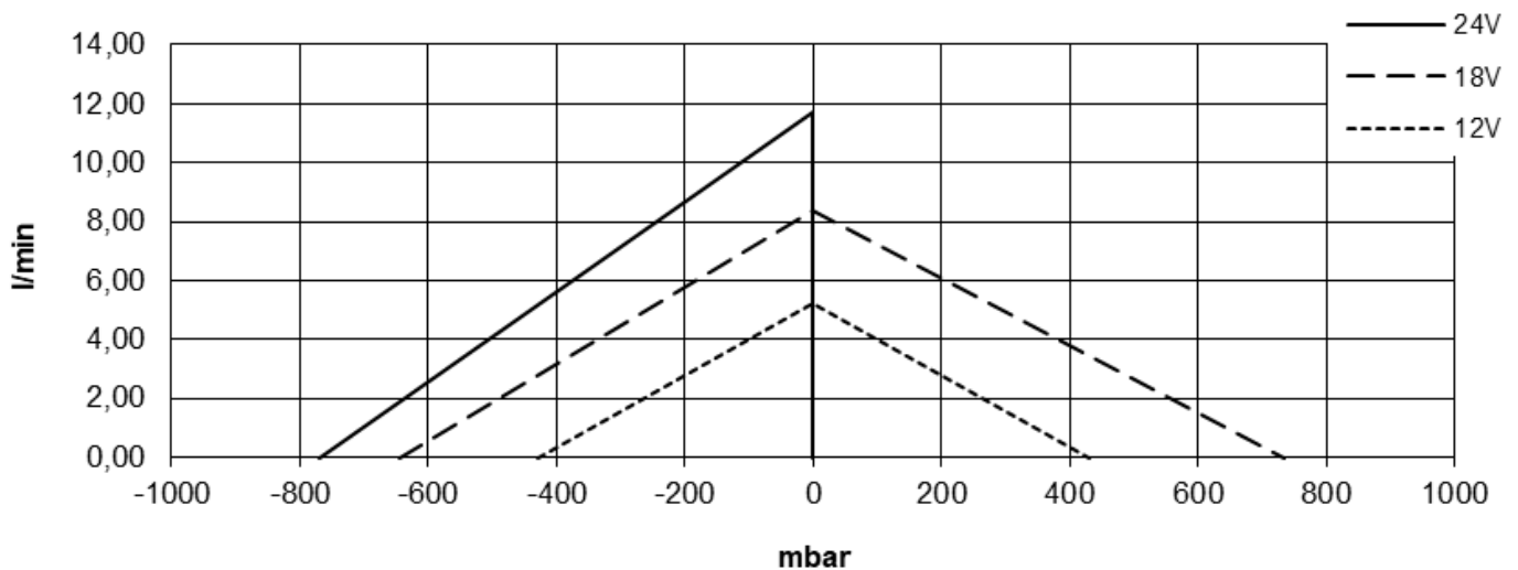
Type/Model: DC24/90KL
